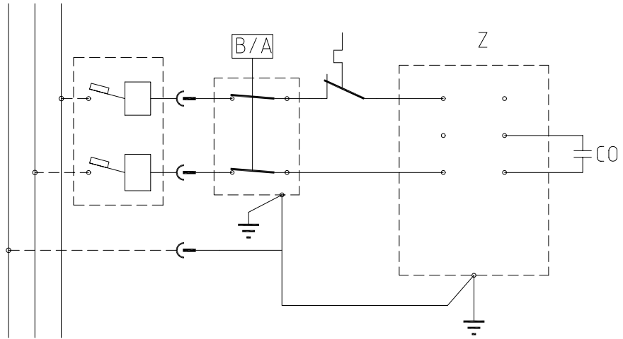
Vienfazē srovē
