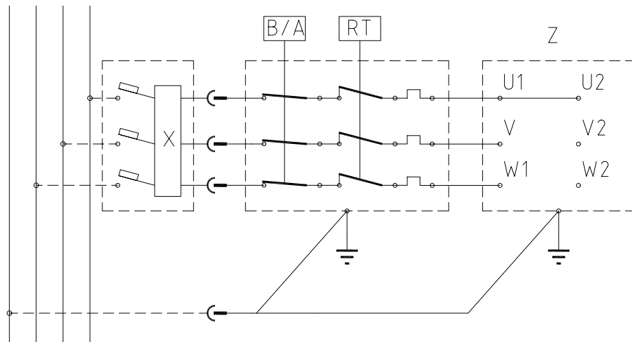
Трёхфазный
