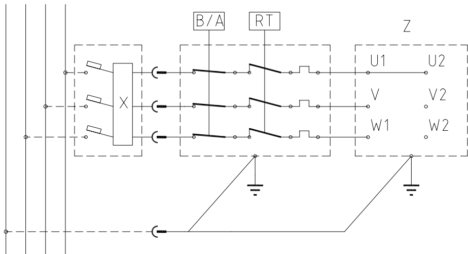
Trifazē srovē
